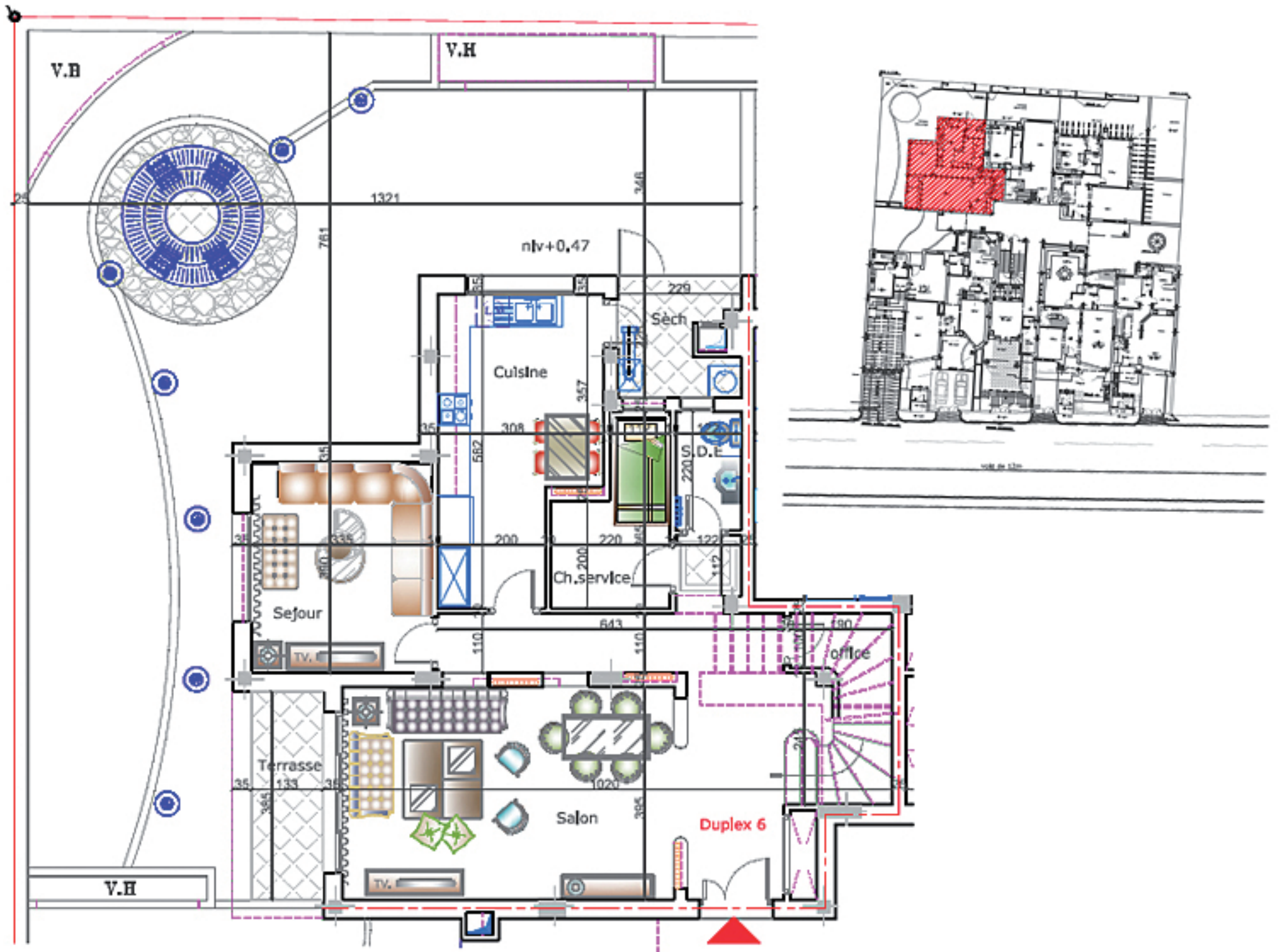
PLAN REZ DE CHAUSSEE
